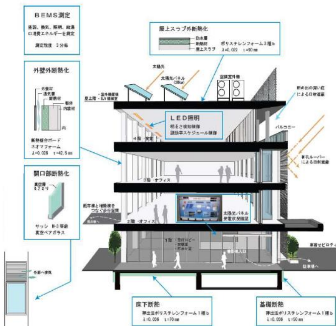
図 アール・ビー・コントロールズ社屋の環境性能
